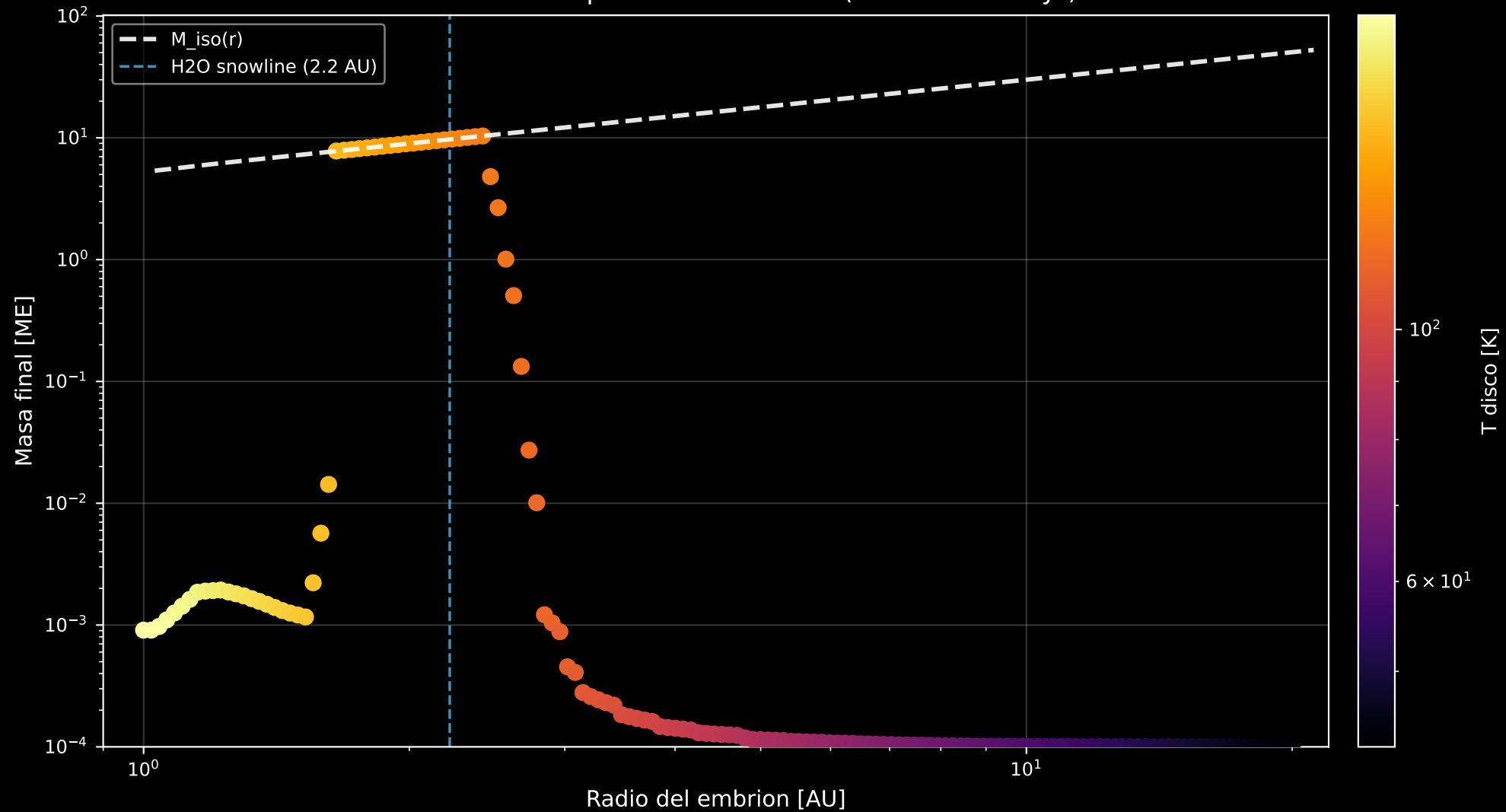
Masa final vs temperatura del disco ( t = 1.00\text{e}+07 yr)
